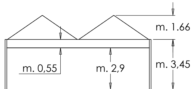
vista laterale
